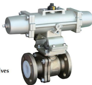
K□PO1159型 衬氟气动球阀 气动操作阀
